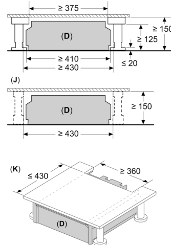
Maße in mm Ansicht von vorne
