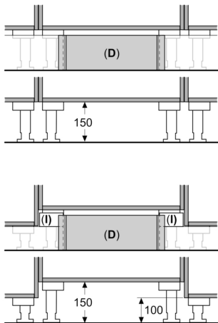
Maße in mm Sockelvarianten für Robotermodul
