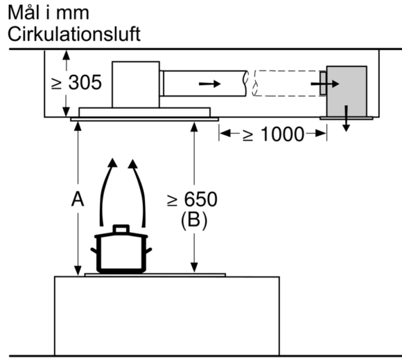
A: Optimal funktion 700-1500 B: Fra overkant af gryderistene
