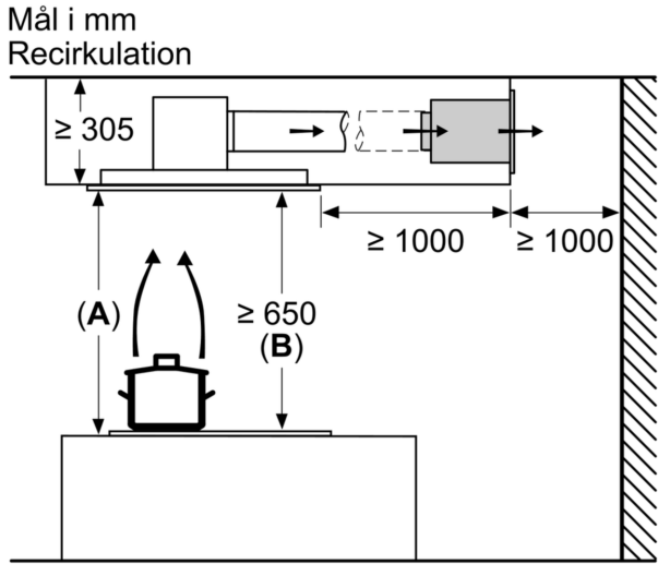
A: Optimal effekt 700-1500 B: Fra overkant af gryderistene
