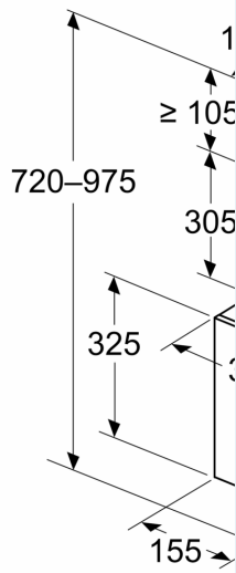
Mål i mm Apparat i recirkulation
