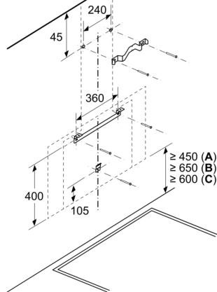
Mål i mm Væginstallation med luftkanal
