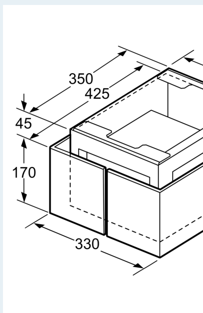
Rozměrové výkresy
