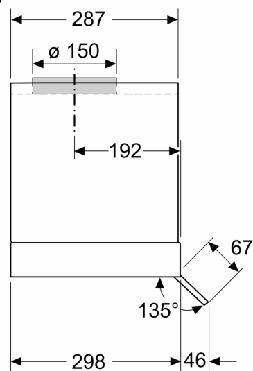
Rozměry v mm Boční pohled
