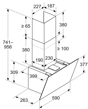
Rozměry v mm Spotřebič v režimu odpadního vzduchu
