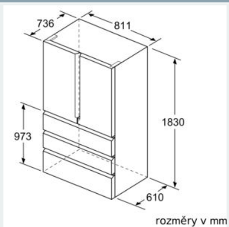
Rozměrové výkresy
