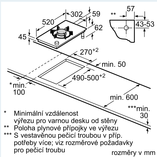
Rozměrové výkresy
