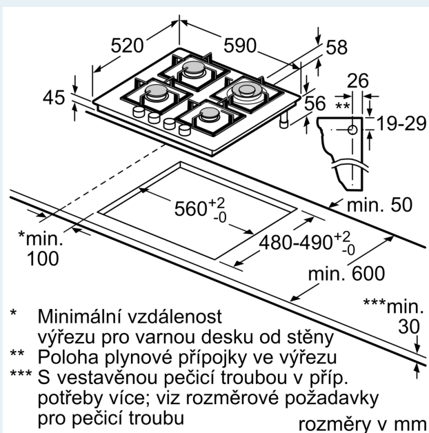
Rozměrové výkresy
