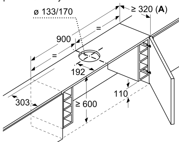
rozměry v mm Upevnění výsuvného odsavače par na závěsný rám
