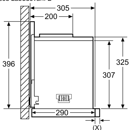
způsob zabudování B
