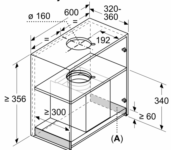
Rozměry v mm Příklad vestavby
