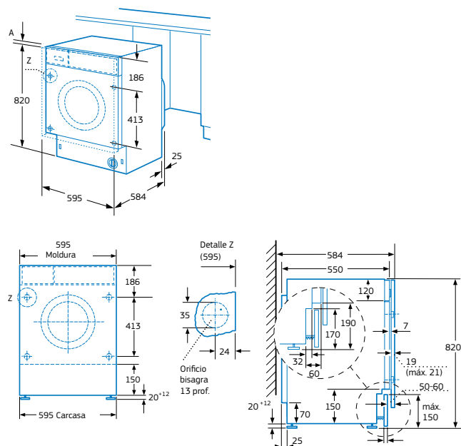
Modelos: 3TI776BC y 3TI773BC
