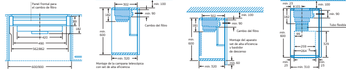
Medidas en mm
