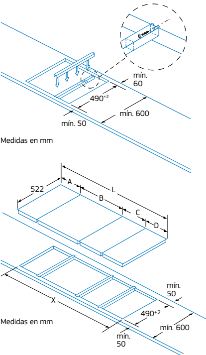
Accesorio de unión 3AB3030L
