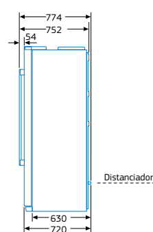
Modelos: 3FA4665X, 3FA4660X y 3FA4611B
