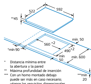
Modelos: 3EB765LQ y 3EB715LR
