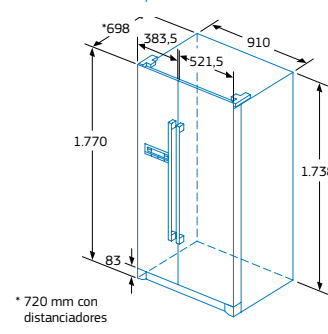
Modelo: 3FA4660X y 3FA4611B
