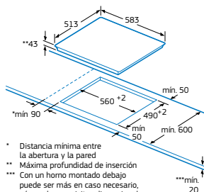
Modelos: 3EB765XQ y 3EB715XR
