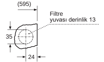
Detay Z
