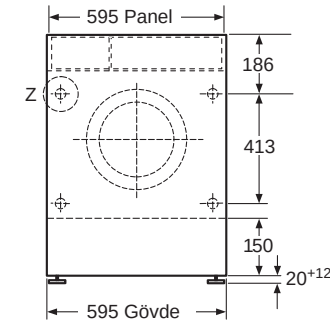
Ölçüler mm cinsindendir
