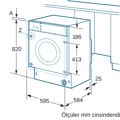
Ölçüler mm cinsindendir
