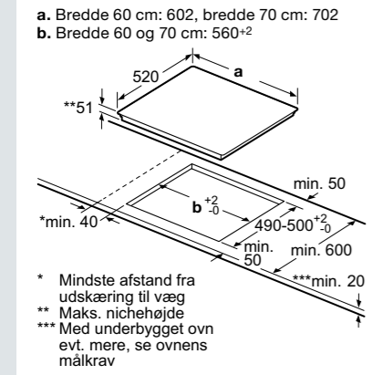
Bredde 60 cm
