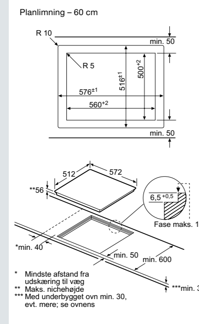
Bredde 60 cm
