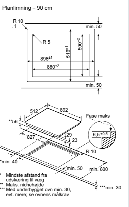
Bredde 90 cm
