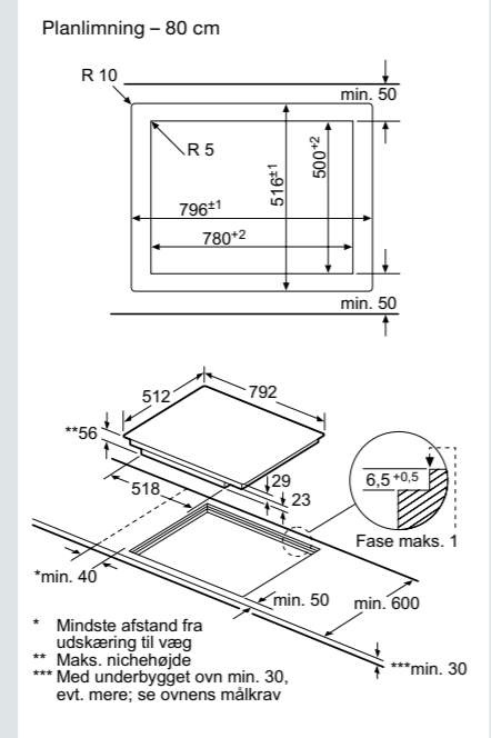
Bredde 80 cm
