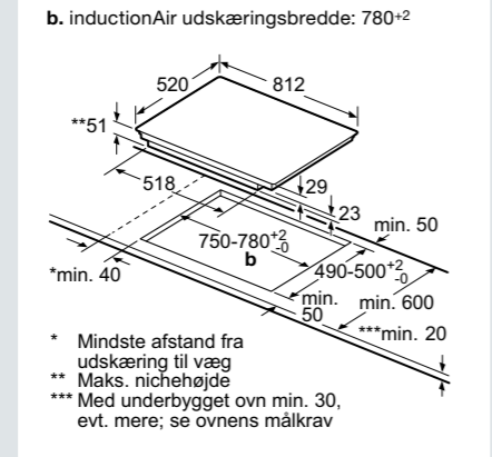
Bredde 80 cm
