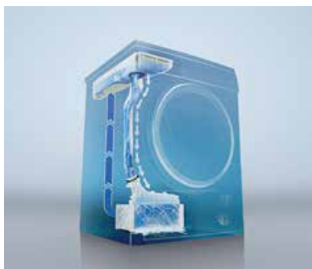
Proceso del condensador autolimpiante.
