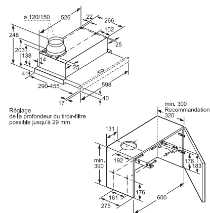
LI64MA520C Dimensions en mm
