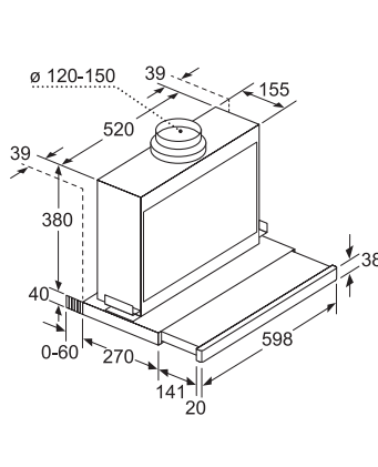
LI26030CH Dimensions en mm
