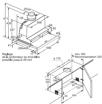
LI67RA560 LI67RA530C Dimensions en mm
