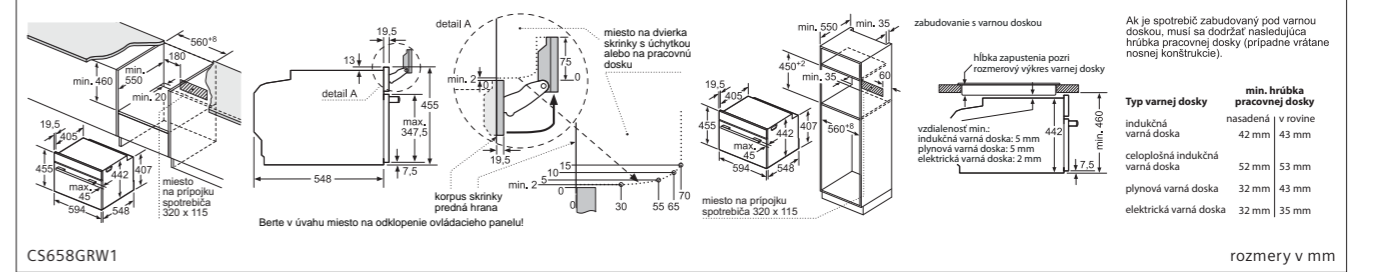
CS658GRW1 rozmery v mm
