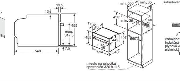
CD634GBW1 rozmery v mm
