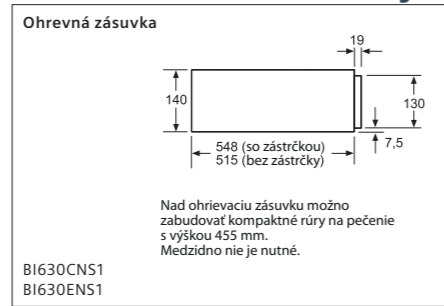
BI630CNS1 BI630ENS1 rozmery v mm
