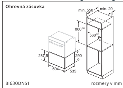
BI630DNS1 rozmery v mm
