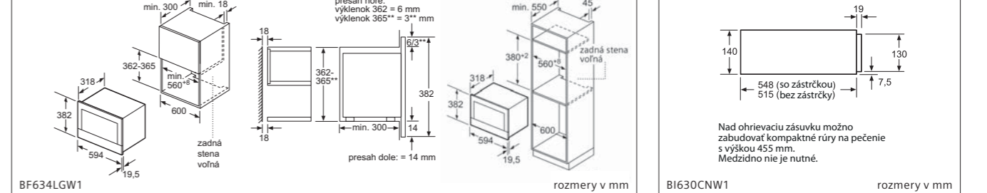
BF634LGW1 rozmery v mm
