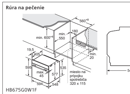
HB675G0W1F rozmery v mm
