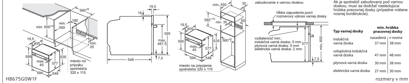
HB675G0W1F rozmery v mm
