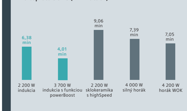
Čas potrebný na ohrev 2 litrov vody s teplotou 15 °C na teplotu 90 °C (v minútach)
