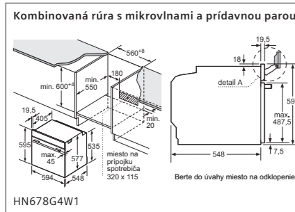
HN678G4W1 rozmery v mm
