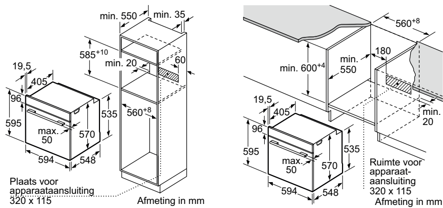
Inbouw met een kookzone.
