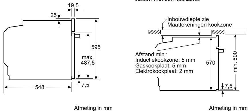
Inbouw met een kookzone.
