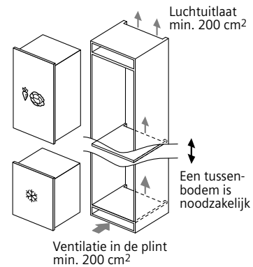
modularFit - Verticale combinatie
