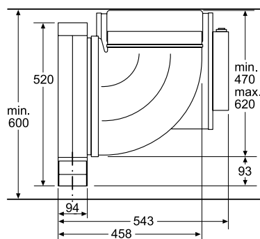
Näkymä yläpuolelta
