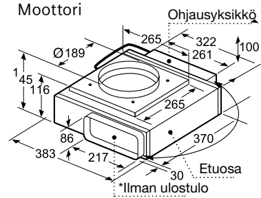
Moottori
