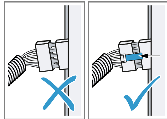
Glasskivans kontakt
