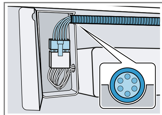
Glasskivans kontakt
