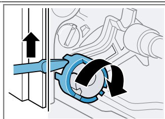
Türsicherung geöffnet
