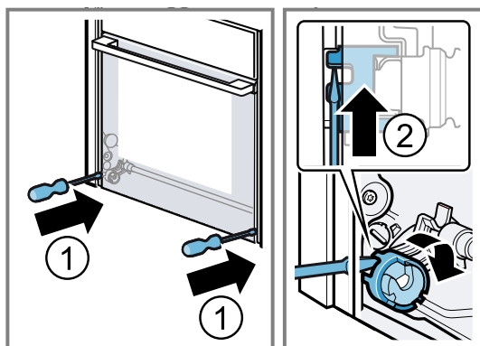
Deurbeveiliging geopend
