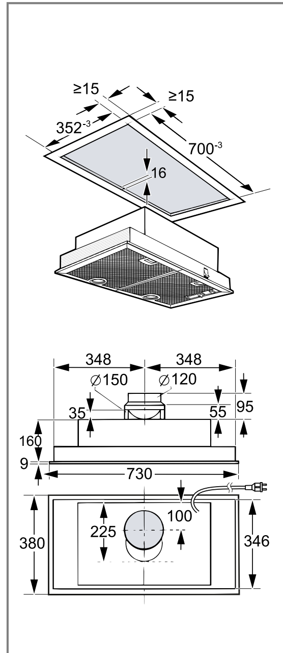
Gerätebreite 730 mm
