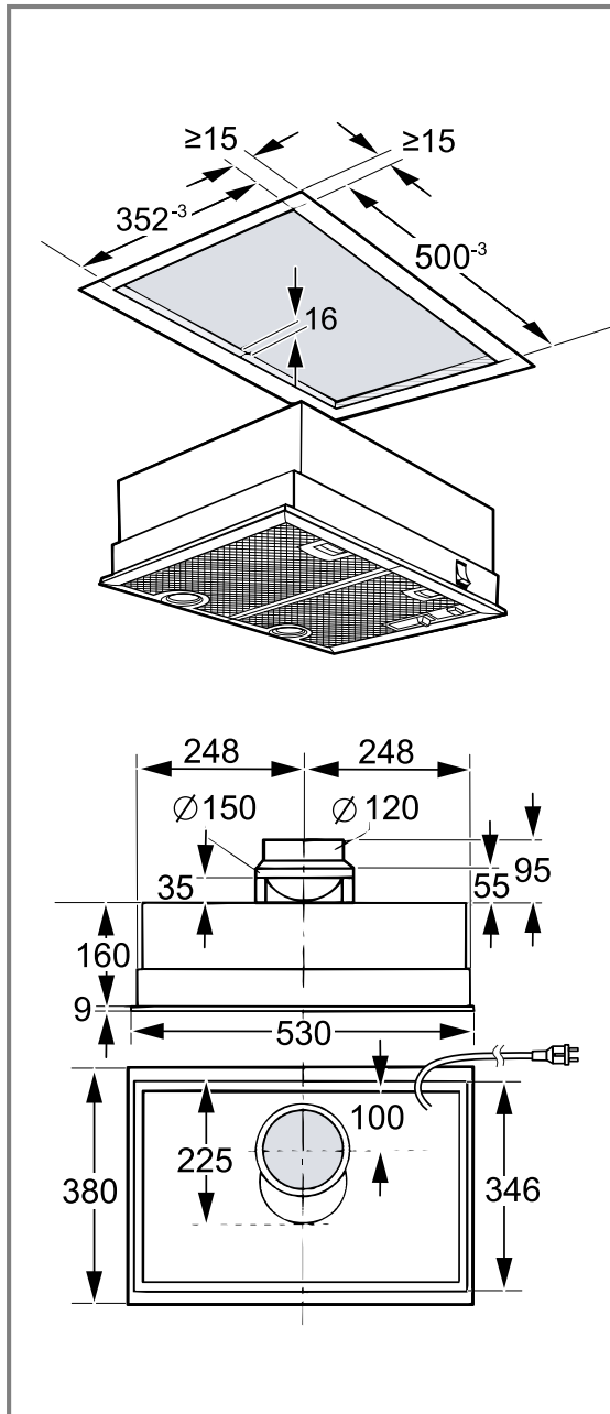
Gerätebreite 530 mm
