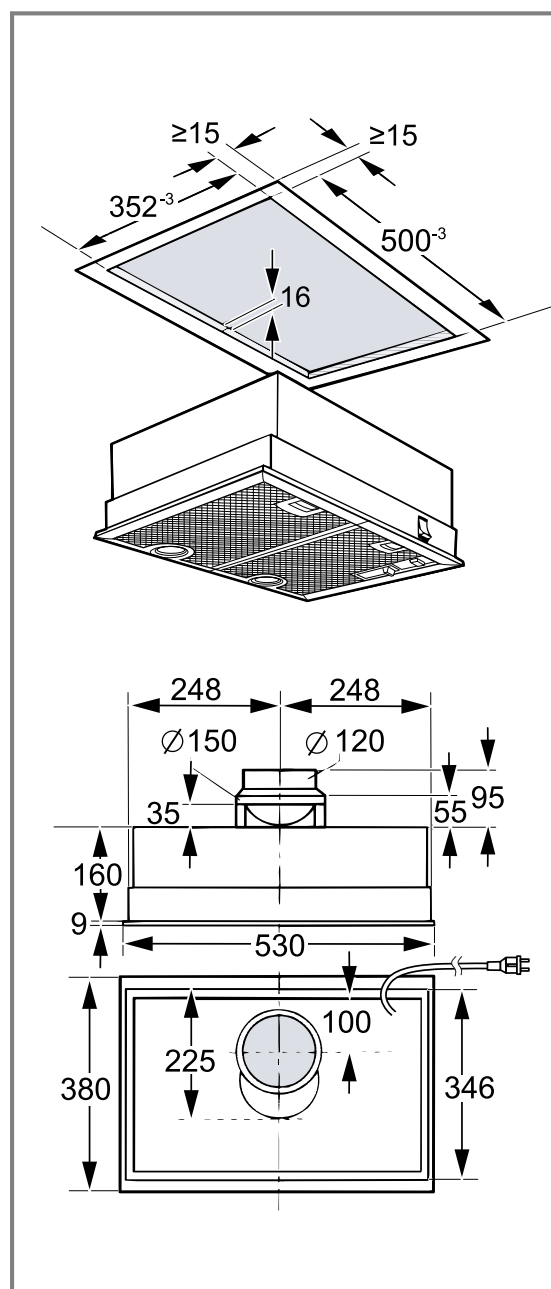
Enhetsbredd 530 mm
