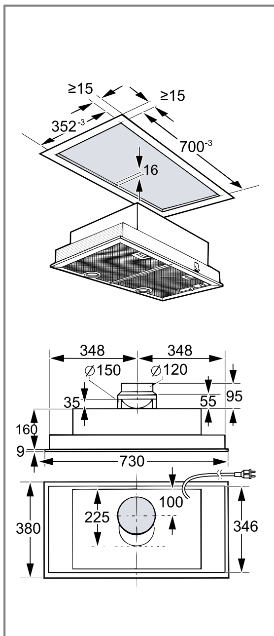
Enhetsbredd 730 mm
