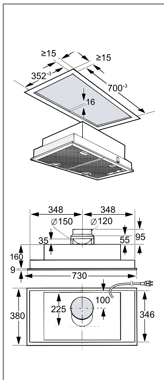
Apparatbredde 730 mm
