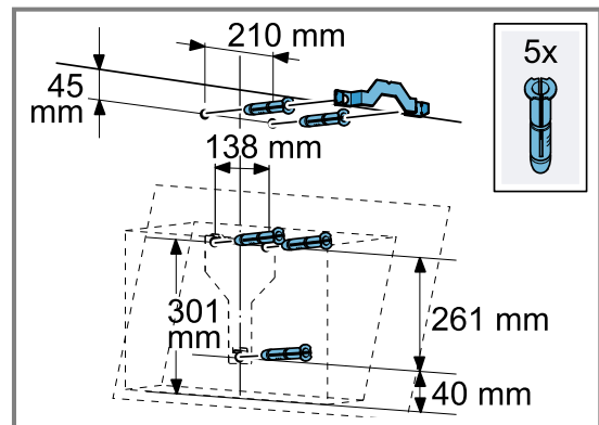
Variant B: schuine afzuigkap met schoorsteenafscherming
