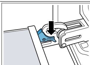
Levier de verrouillage fermé
