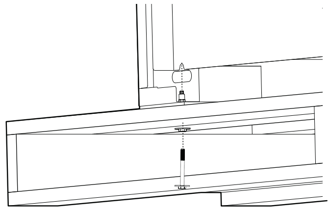
Figure 6 : Retrait des boulons d'expédition
