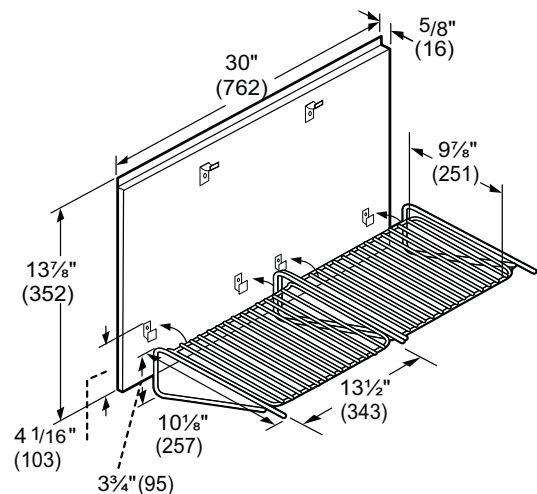
Figura 12: Estante guarda-caliente
