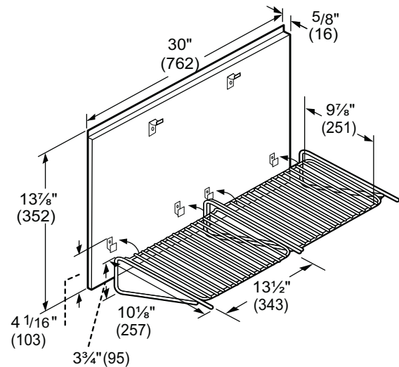
Figure 12 : Étagère garde-chaud
