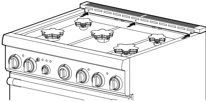
Figura 14: Como quitar los tornillos de la cara frontal
