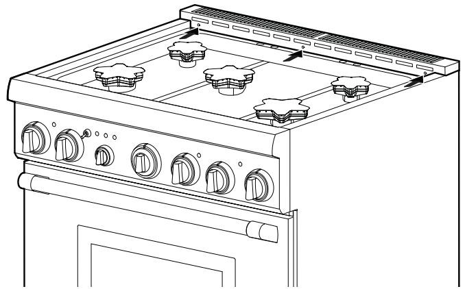
Figure 14 : Retrait des vis de la partie avant
