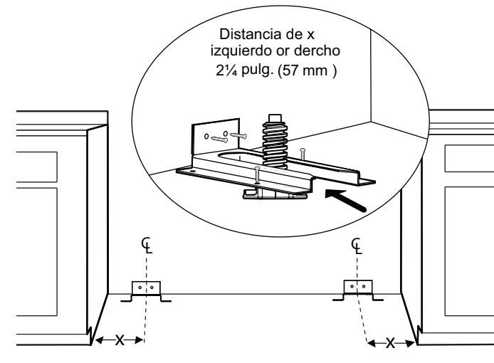
Figura 7: Colocación del dispositivo antivolcadura
