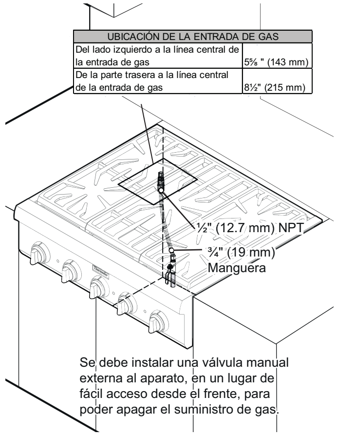
Figura 10: Fondo de unidad
