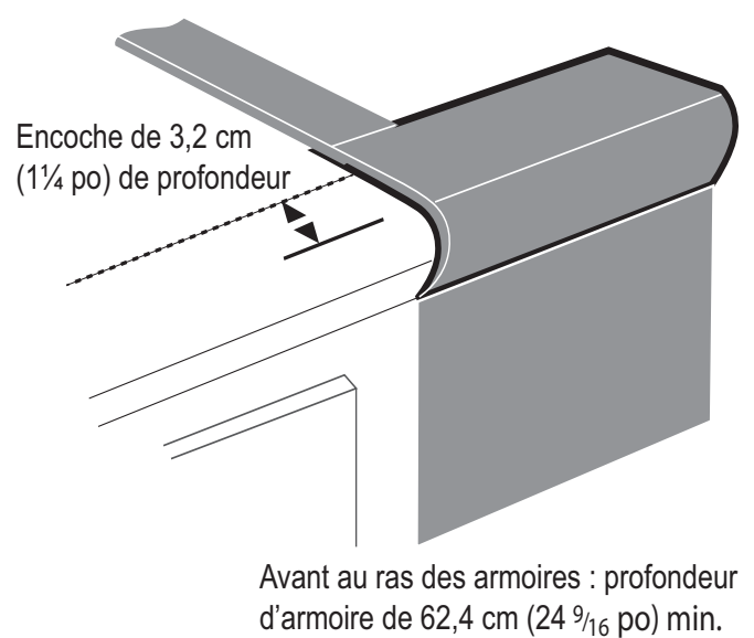
Figure 7 : Au ras du panneau frontal de l'armoire
