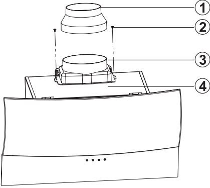
Res. 11: PLASTİK BACA BAĞLANTISI
