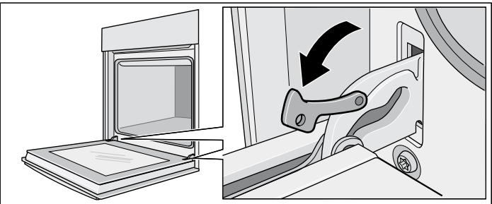
Die Scharniere sind gesichert und können nicht zuklappen.
