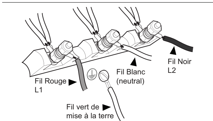
Figure 10 : Connexion à quatre fils
