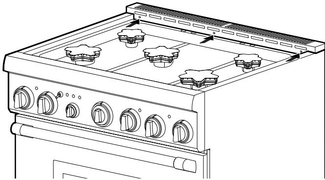
Figura 18: Como quitar los tornillos de la cara frontal
