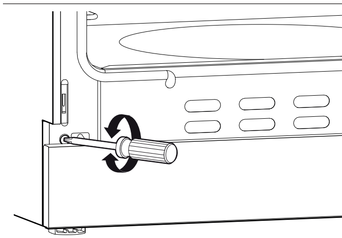
Figura 23: Agujero de los tornillos de ajuste de las bisagras
