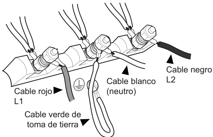
Figura 12: Conexión de 3 cables
