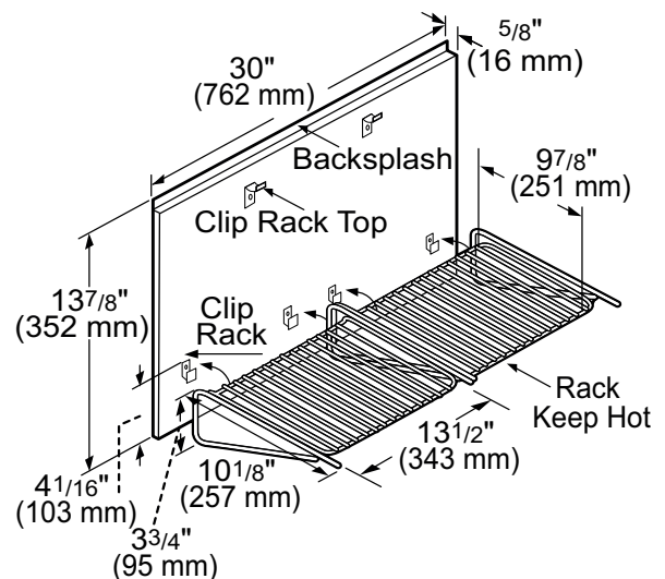
Figure 16 : Étagère garde-chaud
