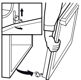
Figura 21: Para quitar la puerta de la hornilla
