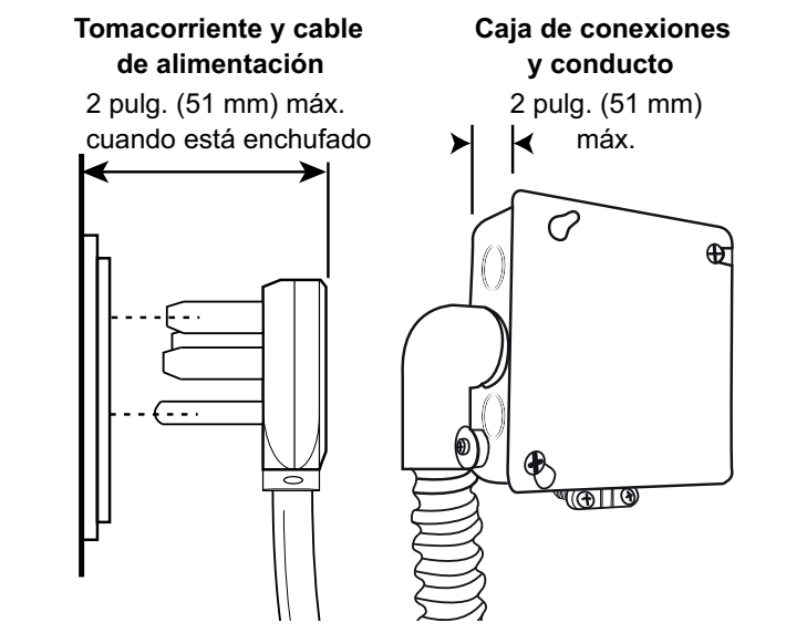
Figura 5: Conexión en la pared
