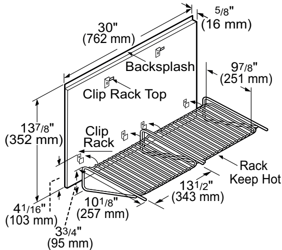
Figura 16: Estante guarda-caliente
