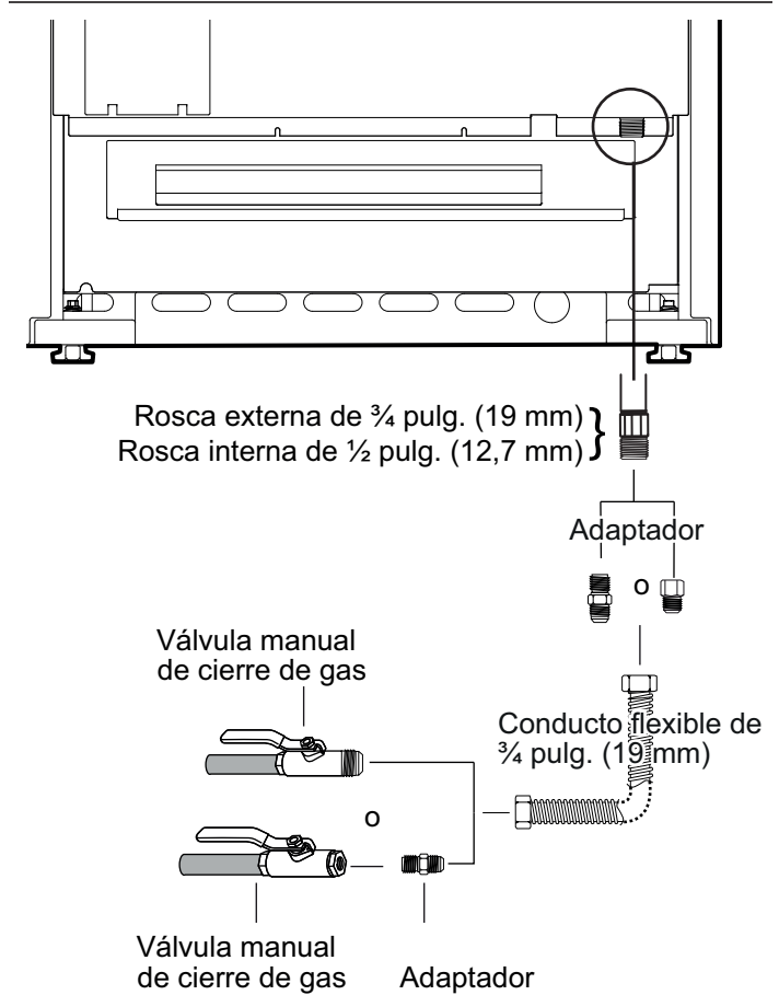
Figura 8: Conexión al suministro de gas
