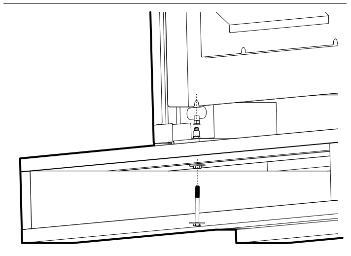
Figura 6: Quitar los pernos de expedición
