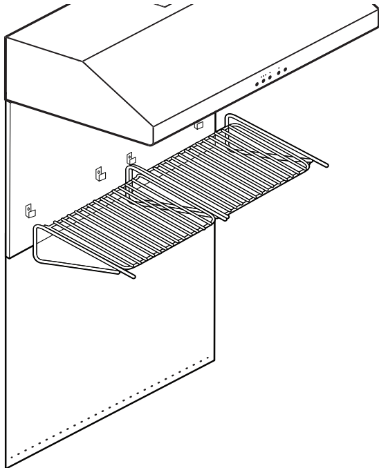
Figura 14: Consola trasera de protección con estante guarda-caliente
