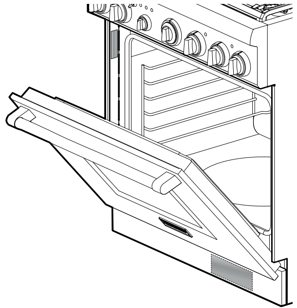
Figure 28 : Emplacement plaque signalétique et diagramme de câblage
