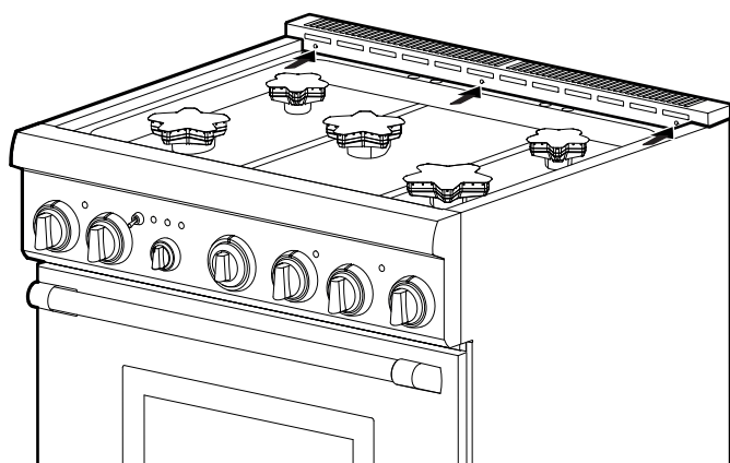
Figure 18 : Retrait des vis de la partie avant
