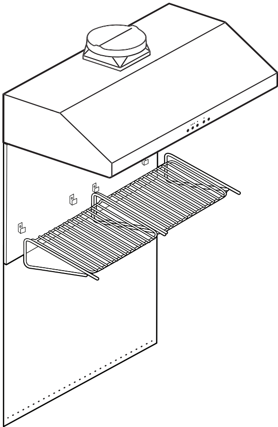
Figure 14 : Dossieret de protection avec étagère garde-chaud
