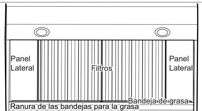
Figura 5: La campana y sus piezas
