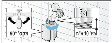
דגם: Aqua-Stop ■
