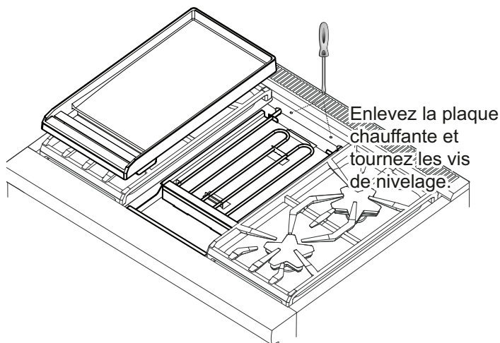
Figure 32 : Vis de nivelage de la plaque chauffante
