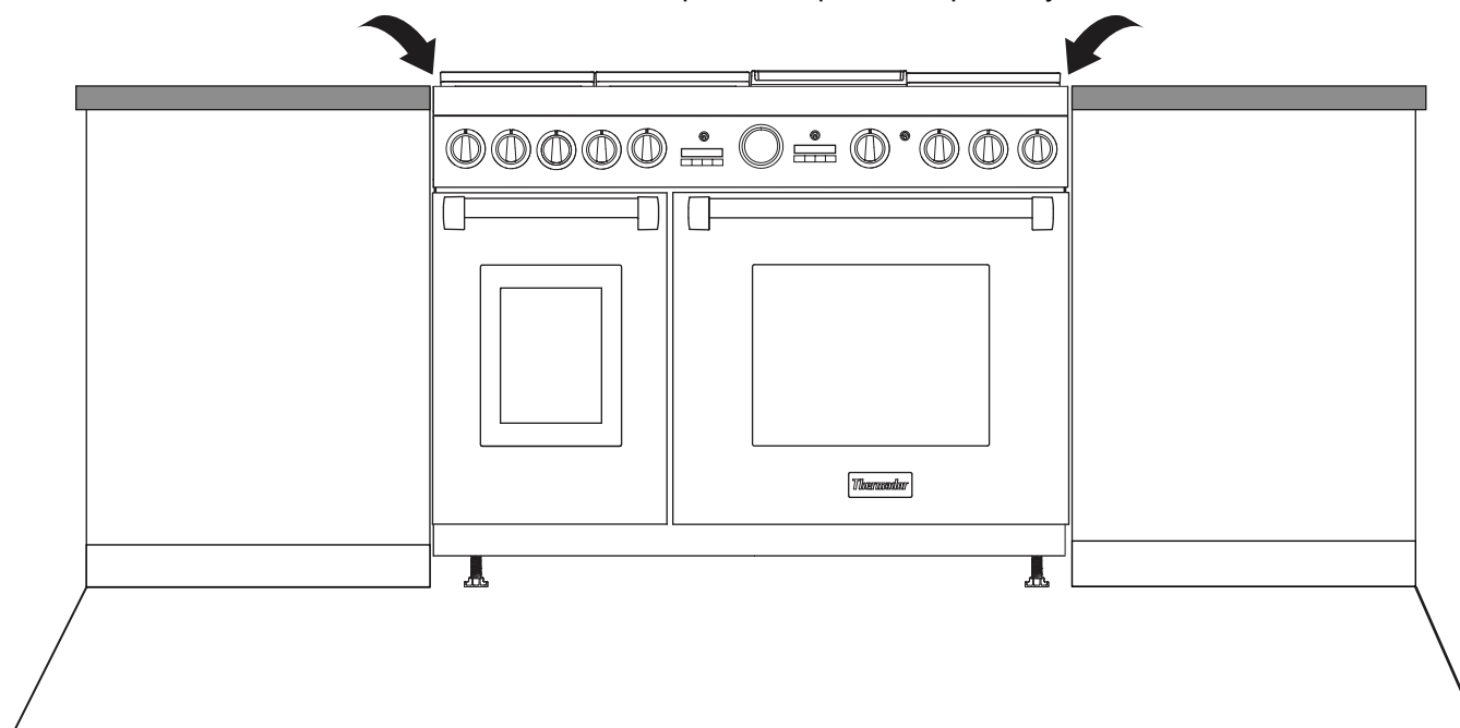
Figure 31 : Réglage de la hauteur de la cuisinière
