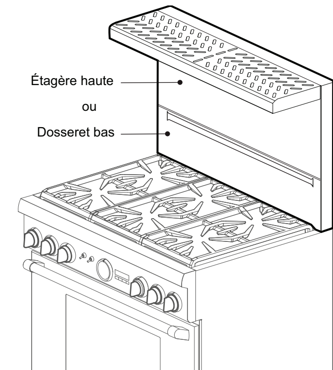
Figure 25 : Vue de face de l'étagère haute et du dosseret bas
