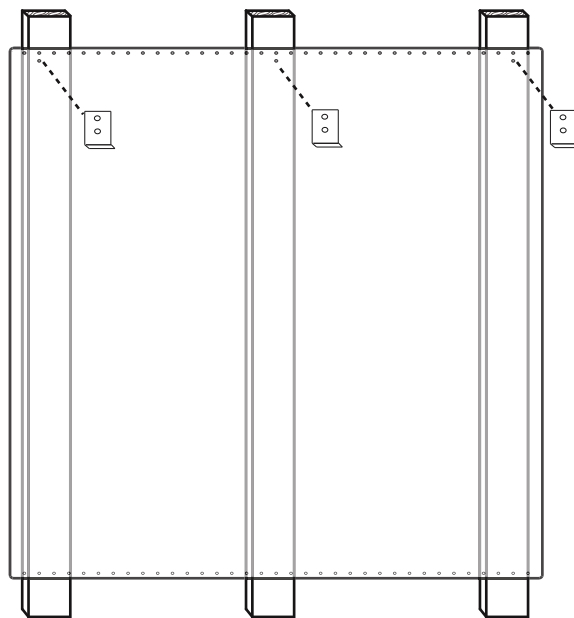
Figure 22 : Dossieret de protection avec étagère garde-chaud
