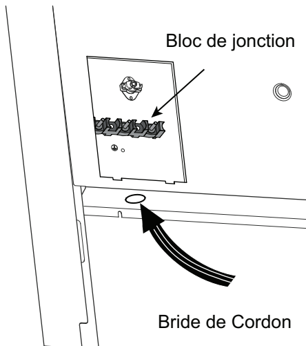
Figure 16 : Emplacement de la bride de cordon
