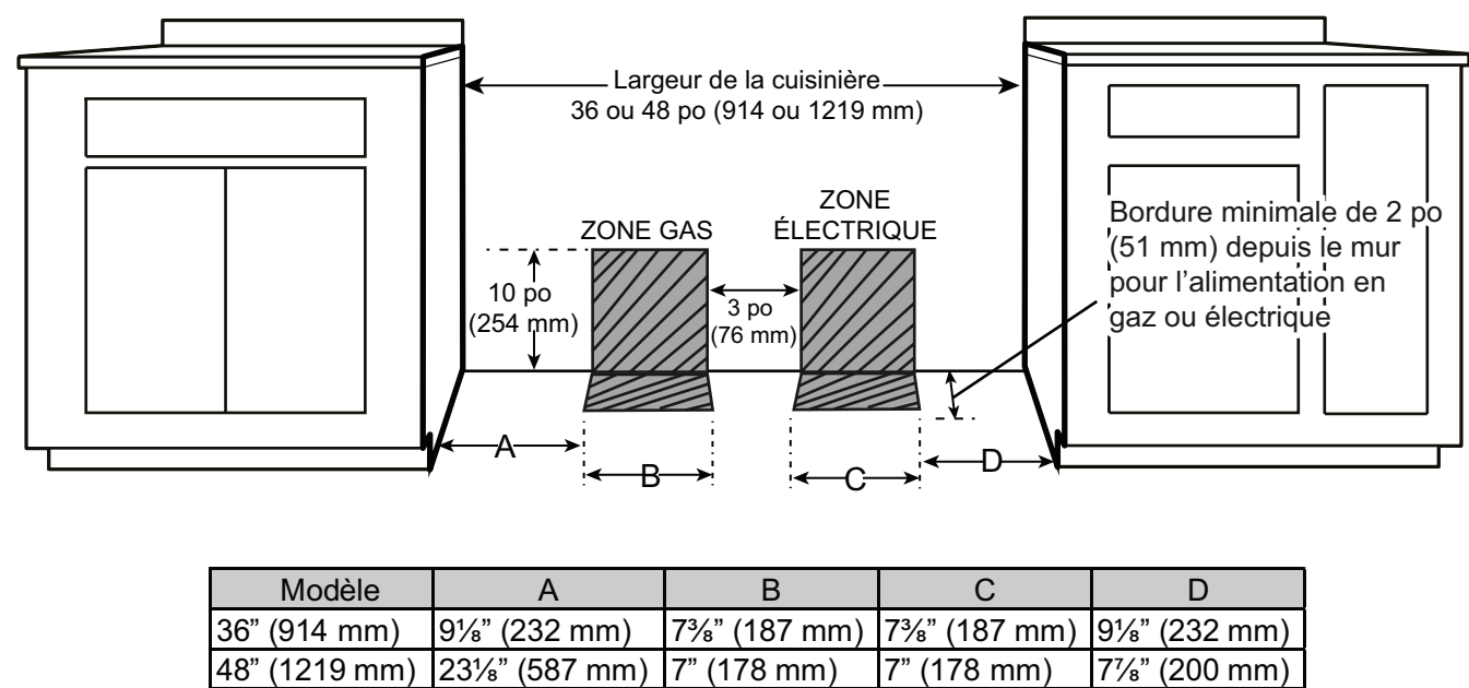
Figure 4 : Emplacement des zones d’approvisionnement en gaz et d’alimentation en électricité
