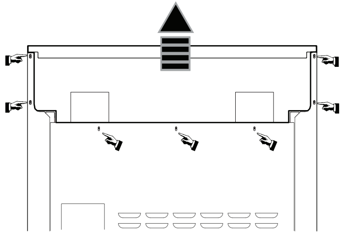
Figura 28: Como quitar los tornillos de la parte trasera del adorno de isla
