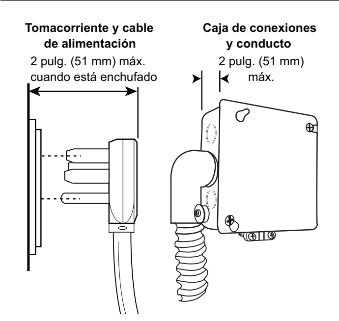
Figura 5: Conexión en la pared
