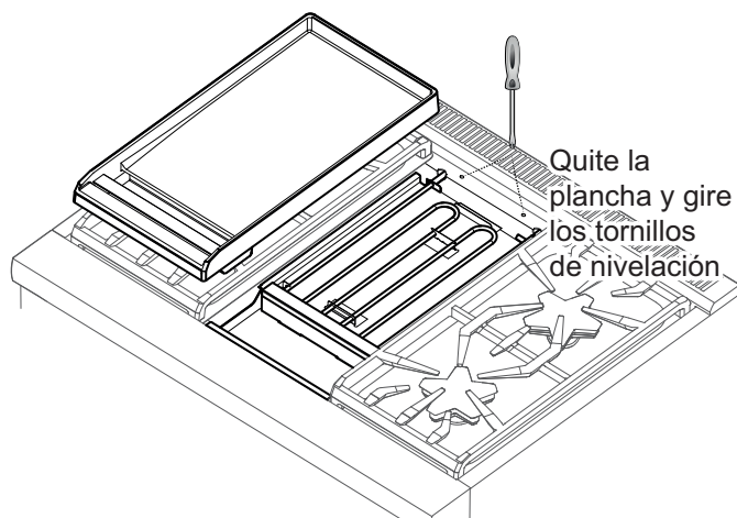
Figura 32: Tornillos de nivelación de la plancha
