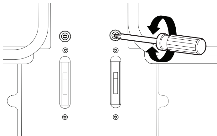
Figure 11 : Vis d'ajustement des charnières
