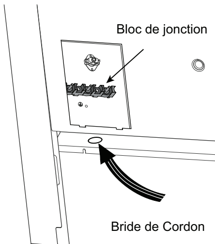
Figure 18 : Emplacement de la bride de cordon
