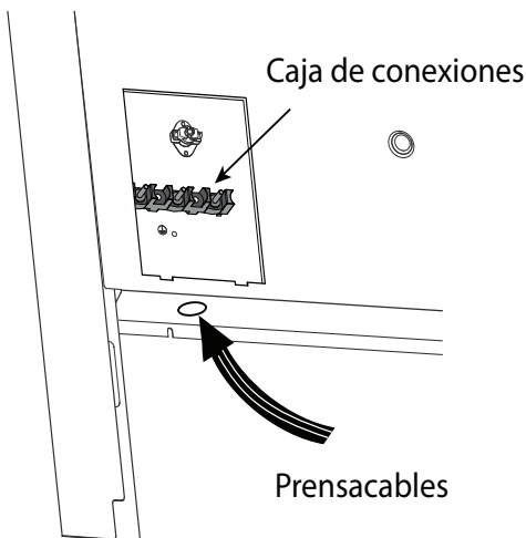
Figura 18: Ubicación del prensacables
