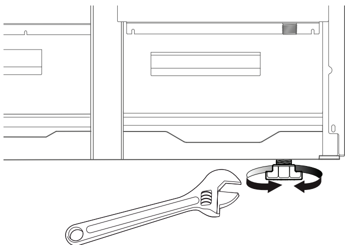
Figure 30 : Ajuster les Pattes
