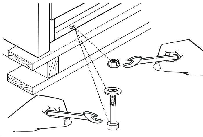
Figure 7 : Enlèvement des boulons de transport
