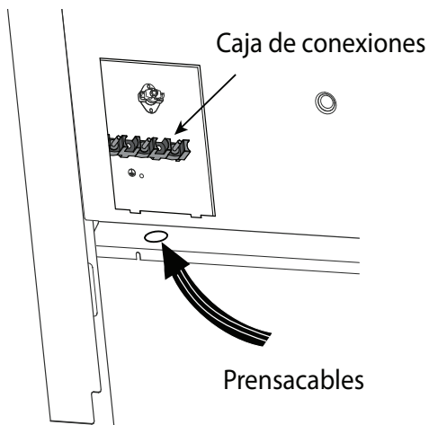
Figura 16: Ubicación del prensacables
