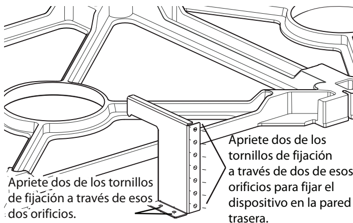
Figura 14: Soporte antivuelco
