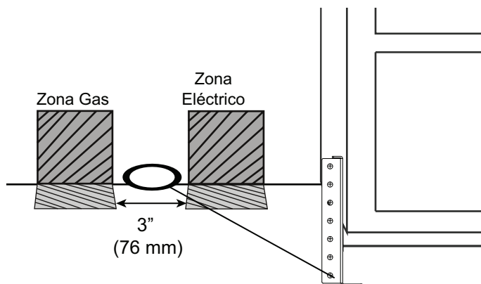
Figura 13: Ubicación para la instalación del dispositivo antivuelco
