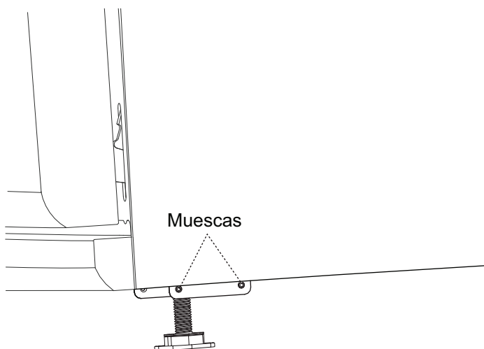
Figura 34: Muecas
