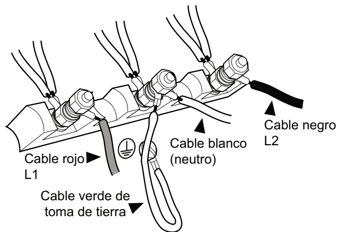
Figura 19: Conexión de 3 cables
