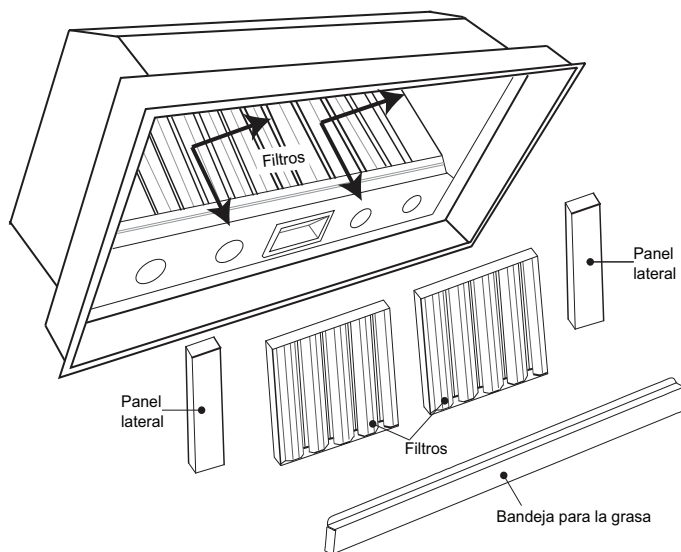
Figura 4: La campana y sus piezas
