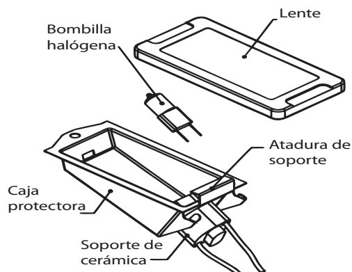
Figura 33: Ensamblaje de la lámpara de la hornilla
