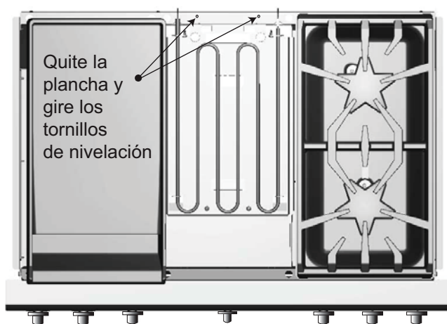
Figura 31: Ajuste de inclinación de la plancha
