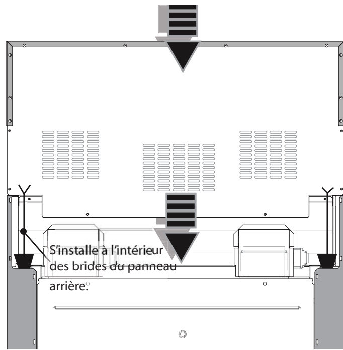
Figure 24 : Installation du dossieret
