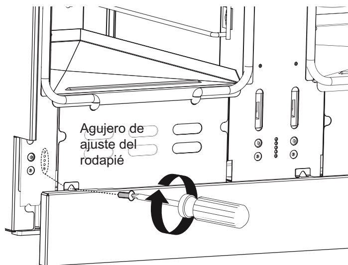
Figura 32: Ajuste del rodapié
