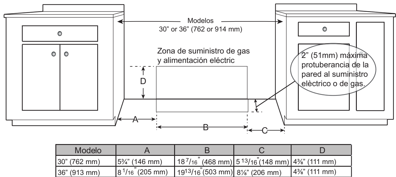
Localización de la conexión de alimentación de gas e eléctrico en estufas de 30" et 36"
