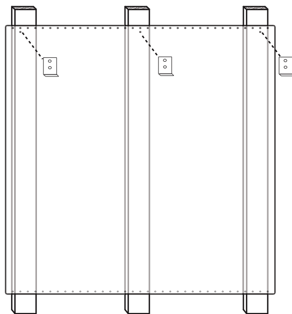
Figura 17: Consola trasera de protección con estante guarda-caliente
