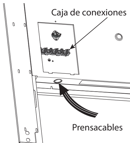
Figura 13: Ubicación del prensacables
