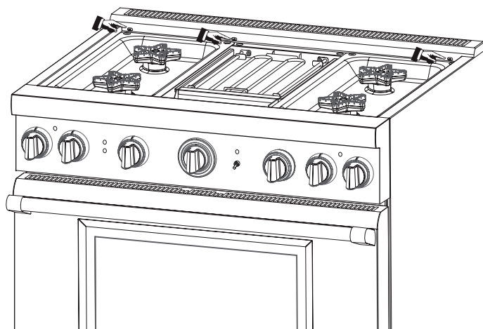
Figure 22 : Retrait des vis de la partie avant de la garniture d'îlot
