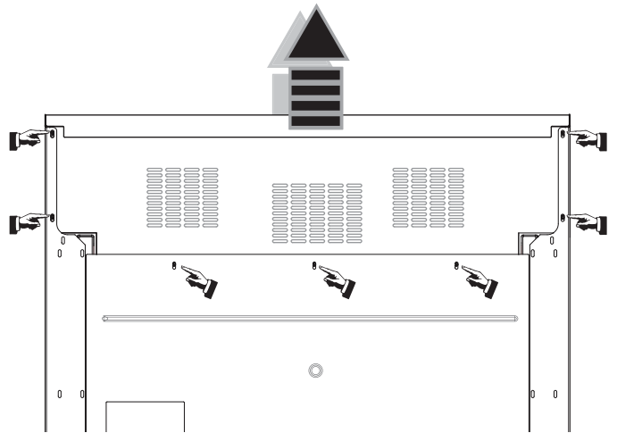
Figura 23: Como quitar los tornillos de la parte trasera del adorno de isla
