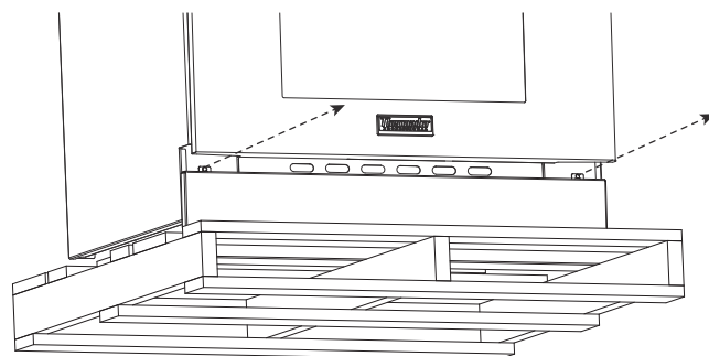
Figure 6 : Retrait du panneau de seuil (plinthe)
