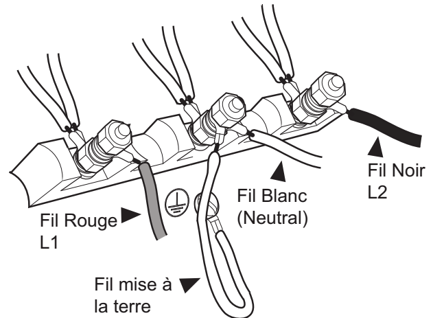
Figure 14 : Connexion à trois fils
