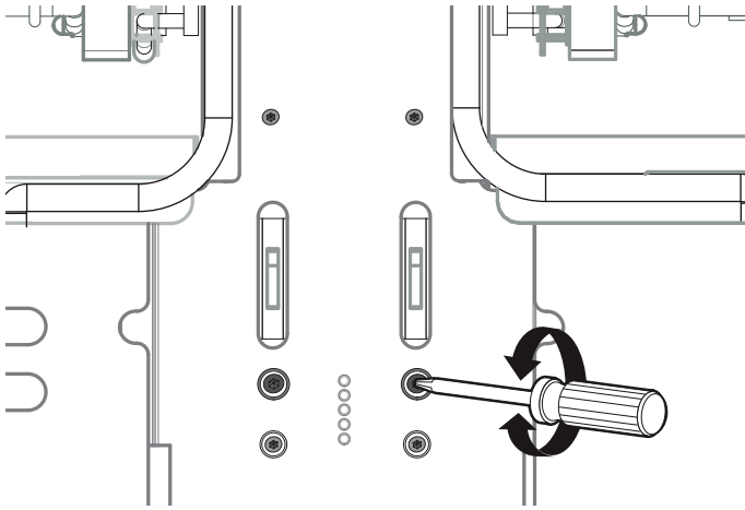
Figura 27: Agujero de los tornillos de ajuste de las bisagras
