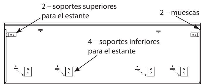
Figura 19: 48 Pulg Dorso de la placa mural
