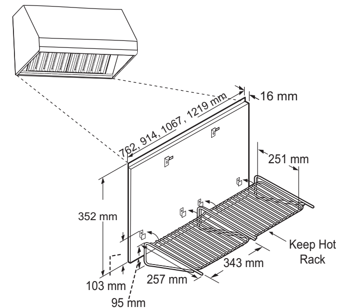
Figura 18: Estante guarda-caliente
