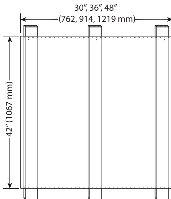
Figure 15 : Installation du dossieret de protection
