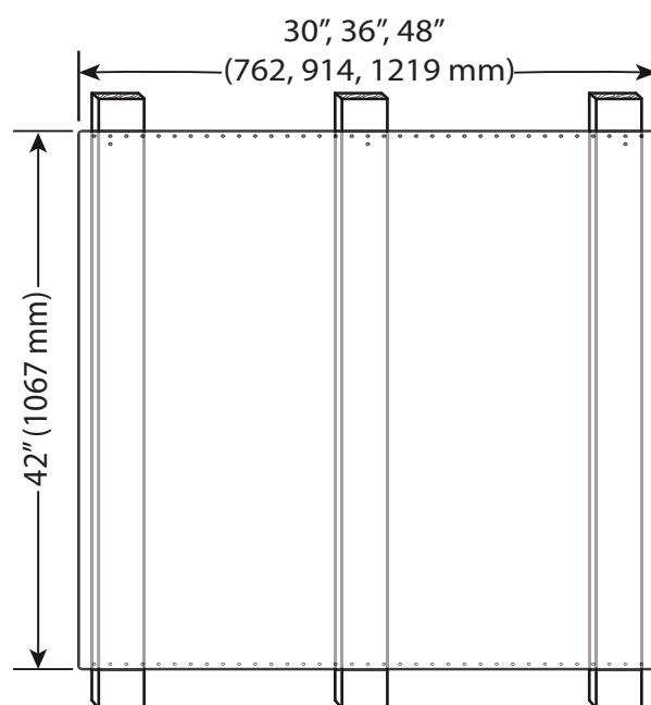
Figura 15: Instalación de la consola trasera
