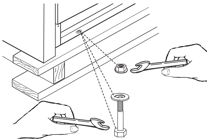
Figure 7 : Enlèvement des quatre (4) boulons de transport
