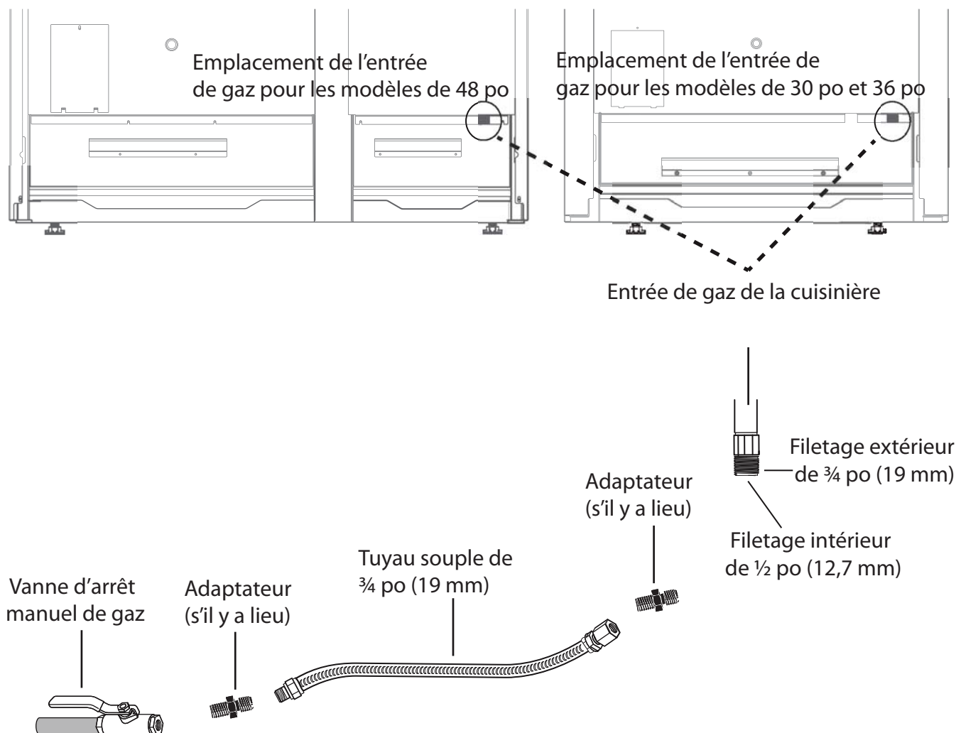
Figure 10 : Raccordement à l'approvisionnement de gaz
