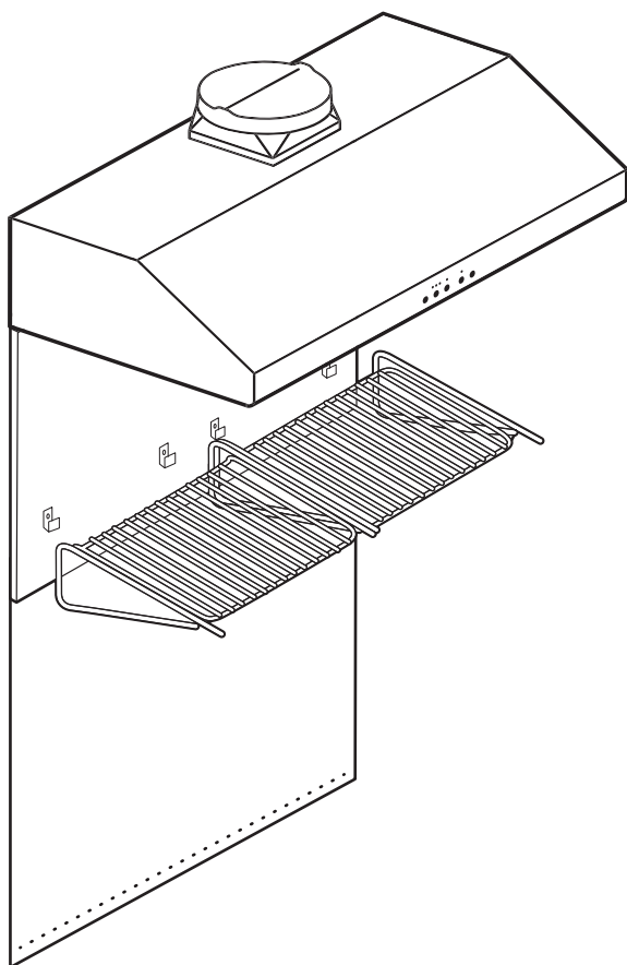
Figure 16 : Dosseret de protection avec étagère garde-chaud
