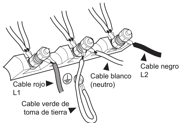
Figura 14: Conexión de 3 cables
