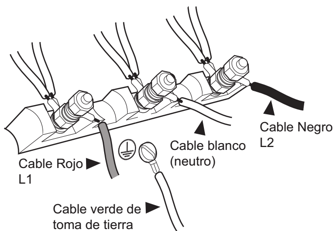
Figura 12: Conexión de cuatro cables
