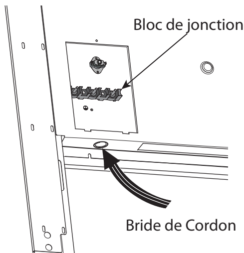
Figure 11 : Emplacement de la bride de cordon
