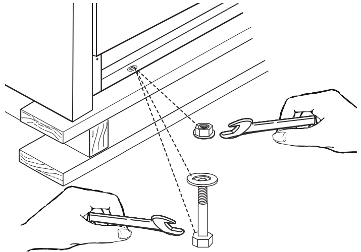
Figura 7: Extracción de los cuatro (4) bulones de transporte
