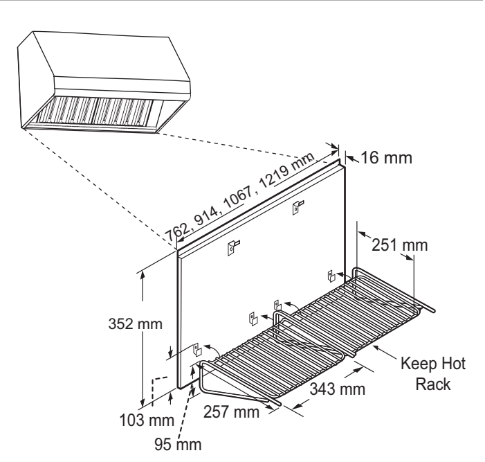
Figure 18 : Étagère garde-chaud
