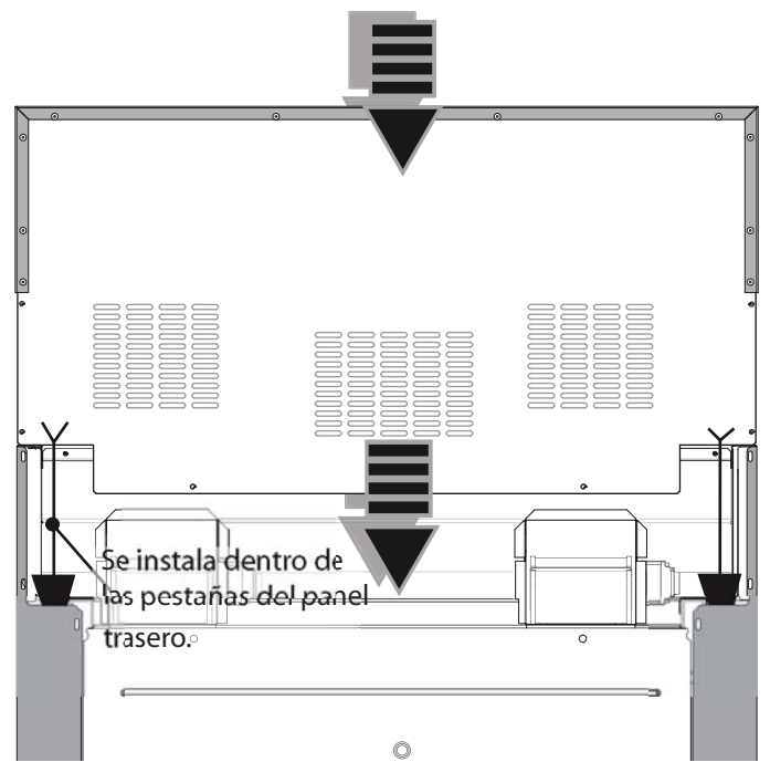
Figura 24: Instalación de la consola trasera baja
