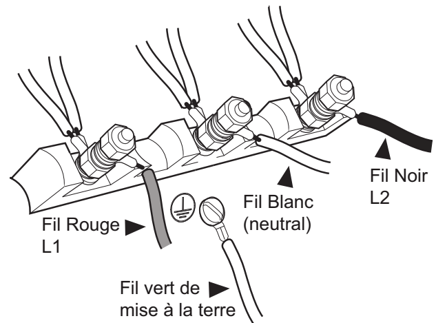
Figure 12 : Connexion à quatre fils
