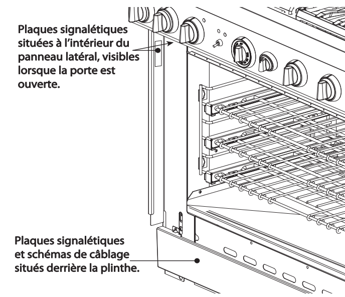
Figure 28 : Emplacement plaque signalétique et diagramme de câblage (porte du four non illustrée)
