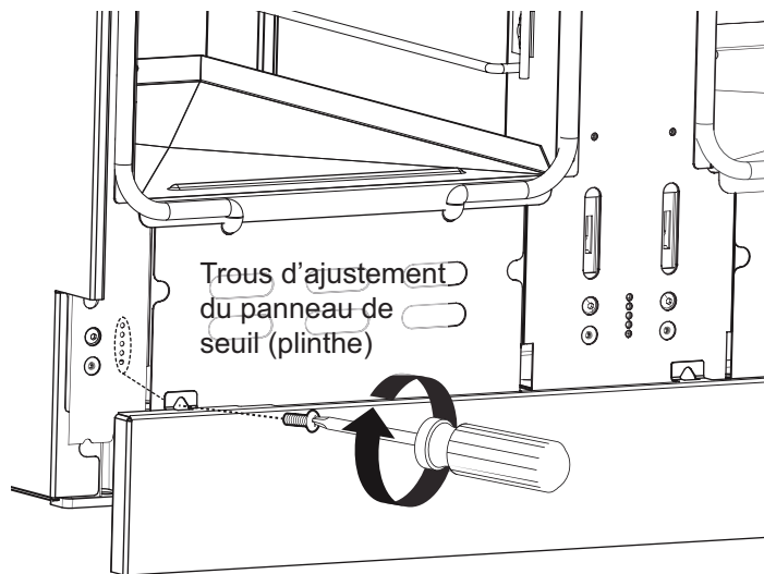
Figure 32 : Ajustement du panneau de seuil (plinthe)
