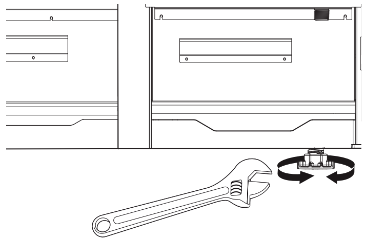
Figure 29 : Ajuster les Pattes
