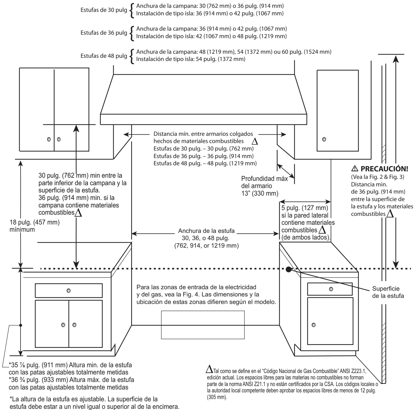
Figura 1: Espacios libres de los gabinetes
