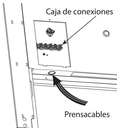
Figura 11: Ubicación del prensacables
