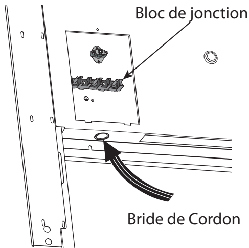
Figure 13 : Emplacement de la bride de cordon
