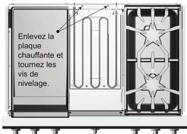
Figure 31 : Vis de nivelage de la plaque chauffante
