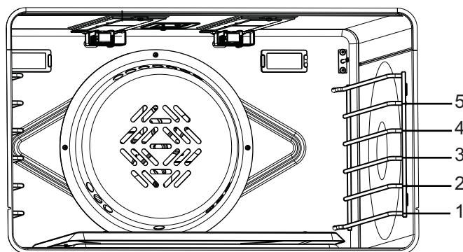
Figura 24: Hornilla principal y posiciones de las rejillas
