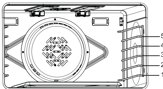
Figure 24 : Four principal au gaz avec positions des grilles
