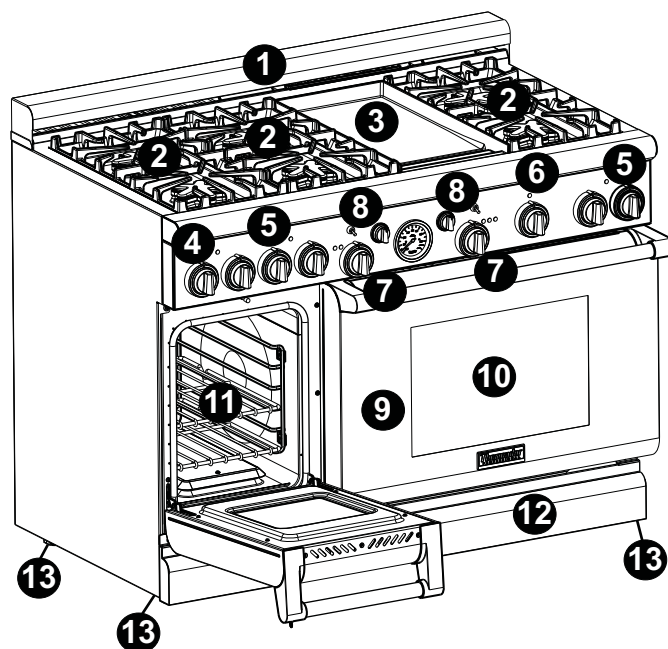
Figura 4: Modelo de 48"
