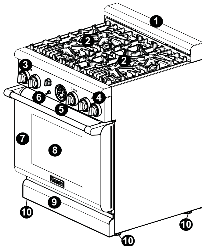
Figura 7: Modelo de 30"
