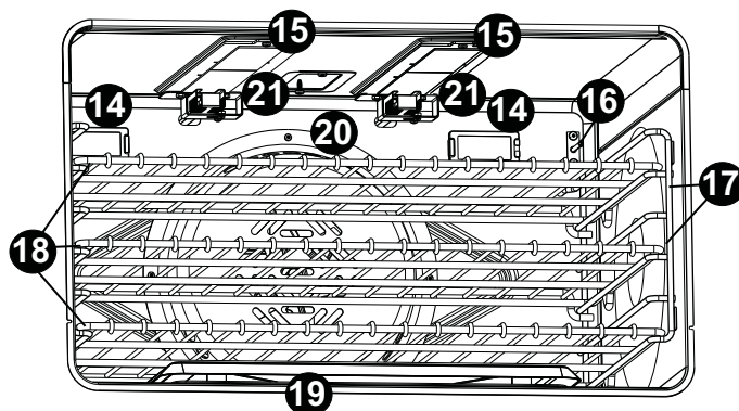
Figure 5 : Intérieur du four au gaz
