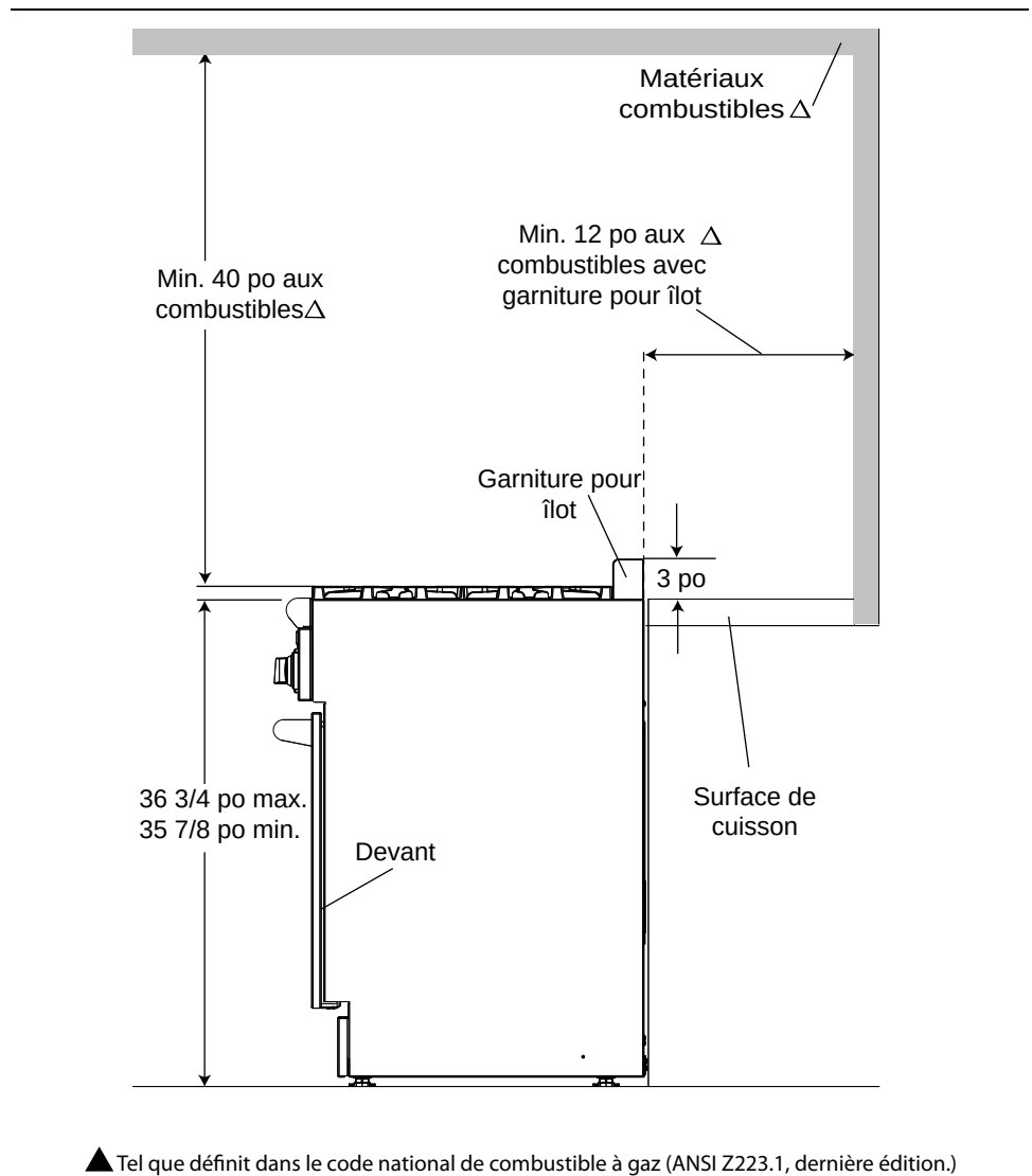
Figure 2b : Vue latérale
