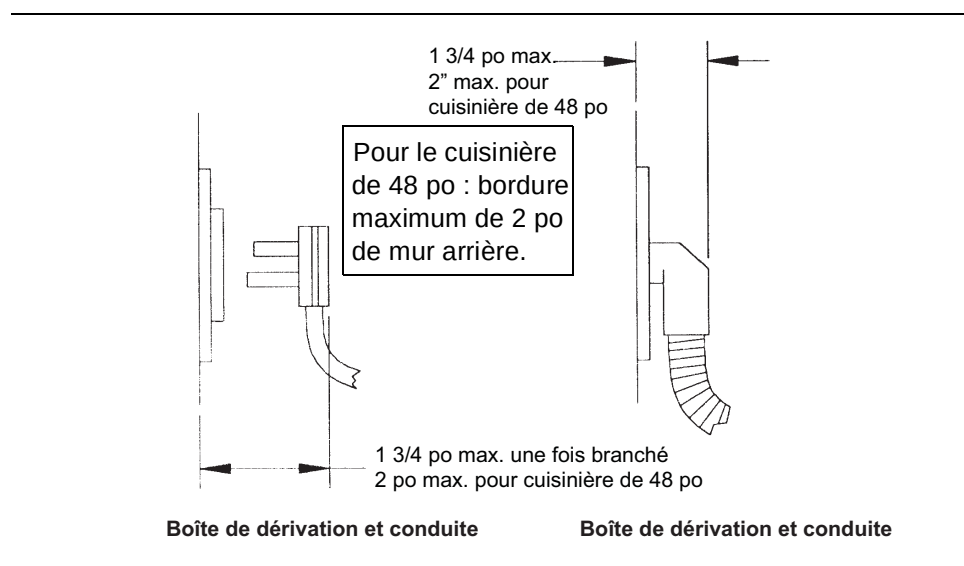
Figure 3b : Raccordement au mur
