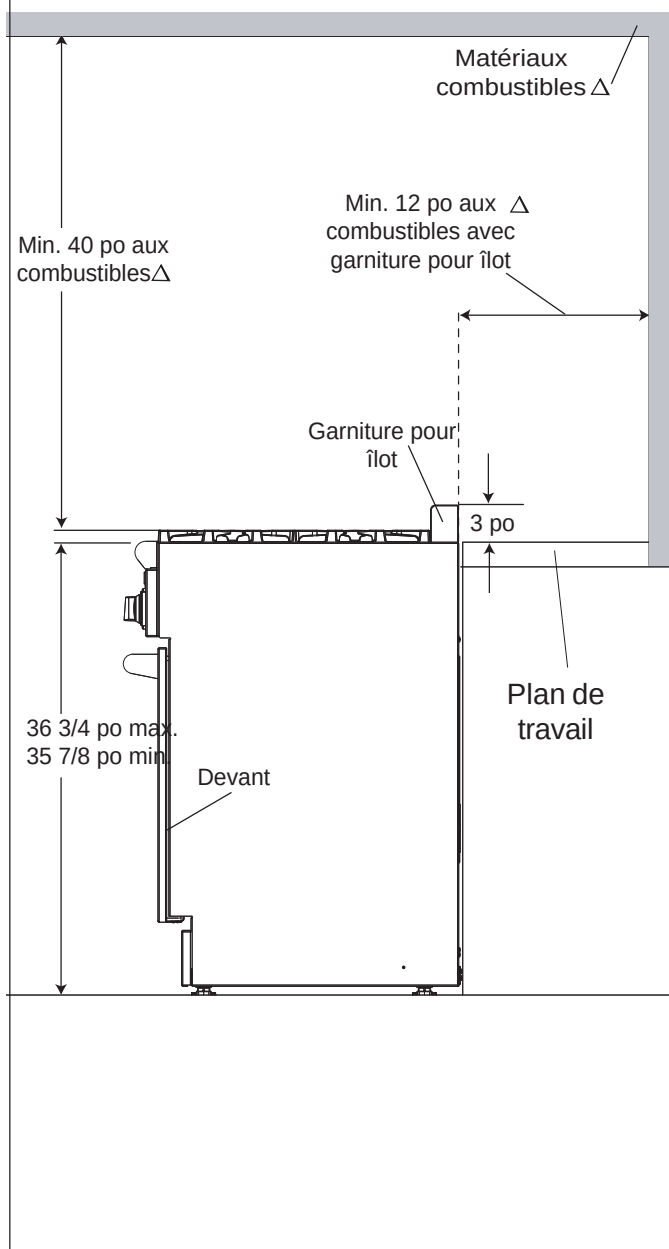
FIGURE 2B - Vue latérale
