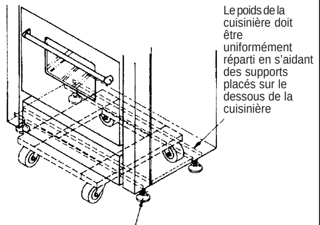
FIG. 5 - Mise en place sur la plate-forme à roulettes
