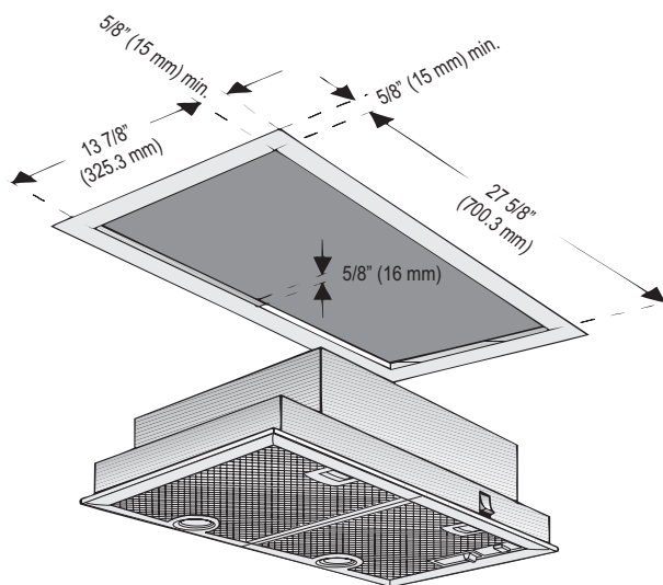
Figure 8: Dimensions de découpes du logement - modèles de 28 3/4 po (73 cm)
