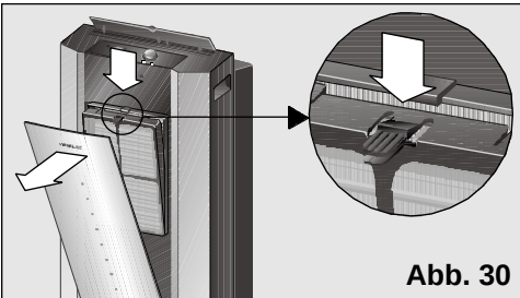
Vlies filter
