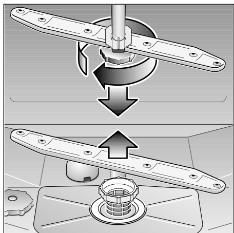
Brazos de aspersión
