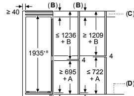
C: Přesah předního panelu
