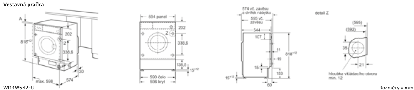
Vestavná kombinace pračka/sušička
