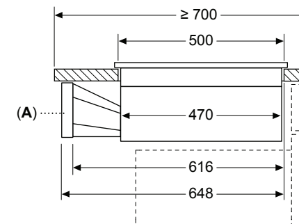
A: Adaptör, yuvarlak-düz
