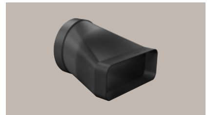
HZ9VDSI0 redukcia na pripojenie plochého potrubia a kruhových prvkov potrubia o Ø 150 mm (samec)
