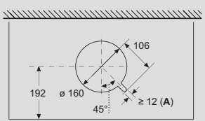
A: Passaggio del cavo
