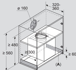
A: Area delle cerniere
