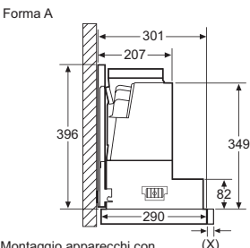
Montaggio apparecchi con telaio di abbassamento - Profondità del mobile secondo la tabella delle combinazioni
