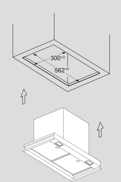
Esempio di montaggio nell'apertura del mobile
