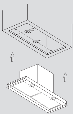
Esempio di montaggio nell'apertura del mobile
