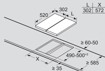
Exemple d'intégration d'un kit d'installation 2 tables de cuisson Domino
