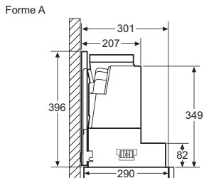
Montage pour les appareils avec cadre d'abaissement. Profondeur du meuble conforme au tableau des combinaisons
