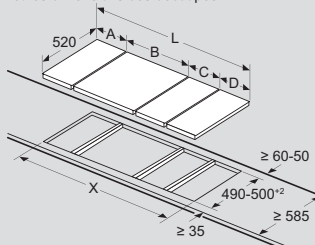
Exemple d'intégration d'un kit d'installation 3 Tables de cuisson Domino + 1 table de cuisson
