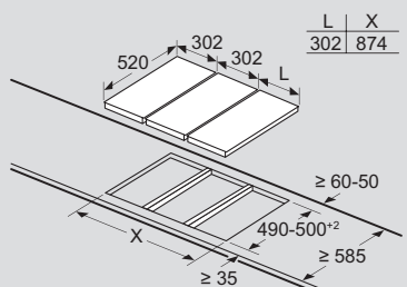
Exemple d'intégration d'un kit d'installation 3 tables de cuisson Domino
