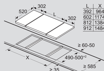
Exemple d'intégration d'un kit d'installation 2 Tables de cuisson Domino + 1 table de cuisson
