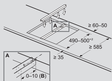
Kit d'installation (HZ394301) pour Domino
