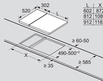
Exemple d'intégration d'un kit d'installation 1 table de cuisson Domino + 1 table de cuisson
